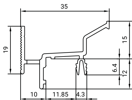
RD 19 K Stil
