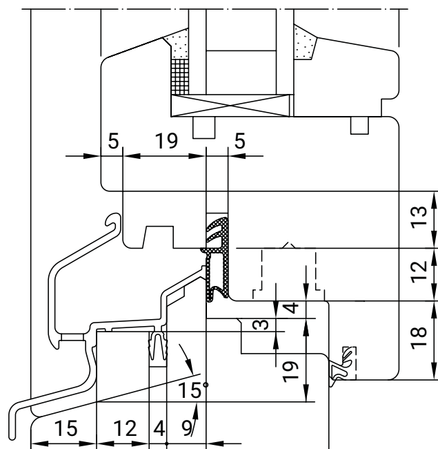
Einbaubeispiel RD 19.45 K
