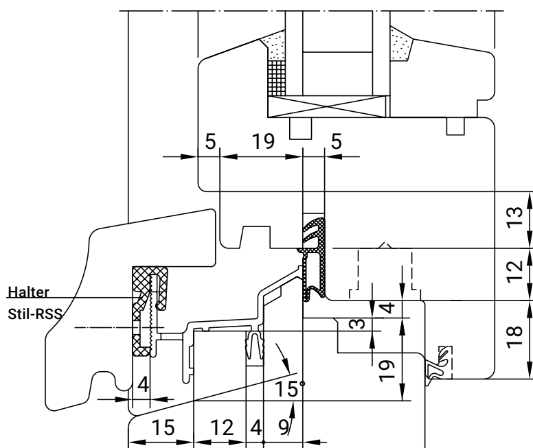
Einbaubeispiel RD 19 K Stil
